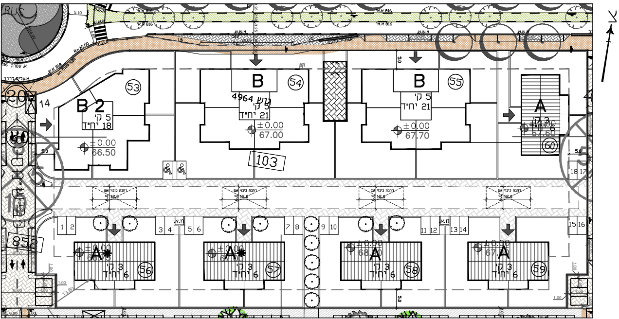
תכנית מגרש מס' 103 ק.מ. 1:1000
