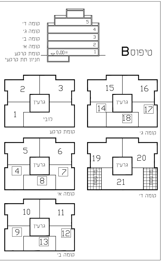
סכמת התפלגות יחיד בבנינים מס' 55.54 18 יחיד קטנות ב 2 בנינים
