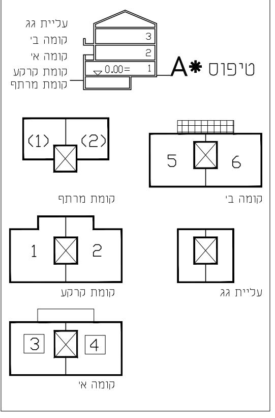
סכמת התפלגות יחיד בבנינים מס' 57.56 4 יחיד קטנות ב 2 בנינים
