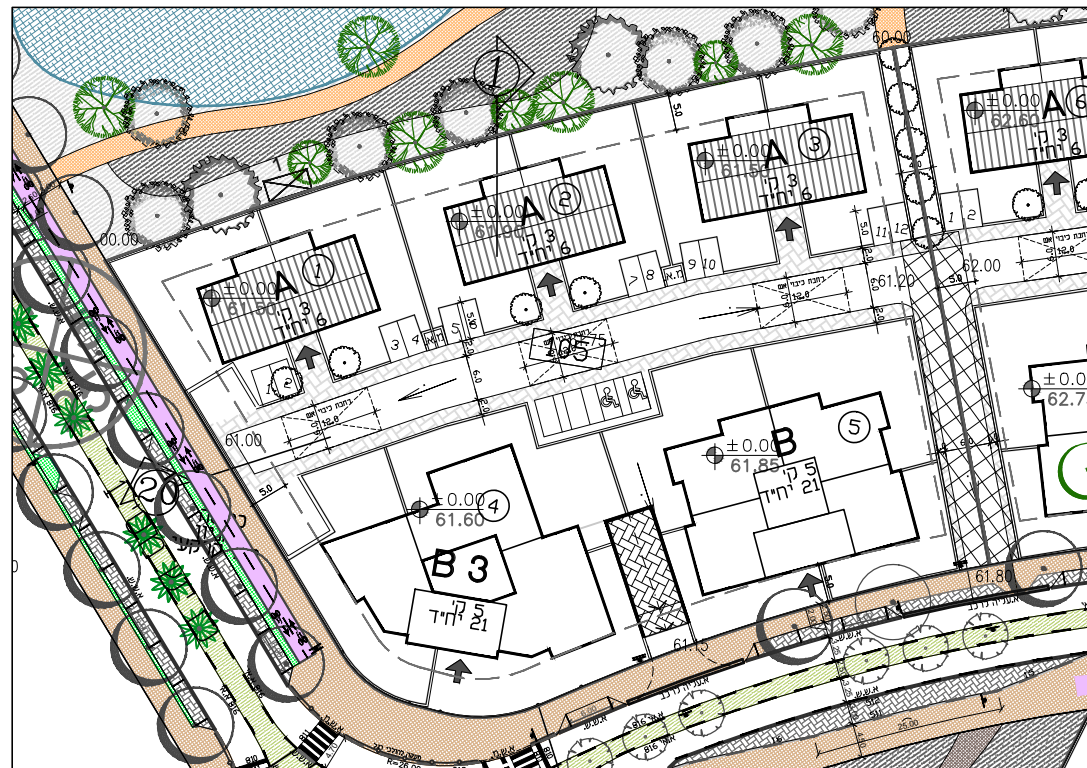
תכנית מגרש מס' 105 ק.מ. 1:1000
