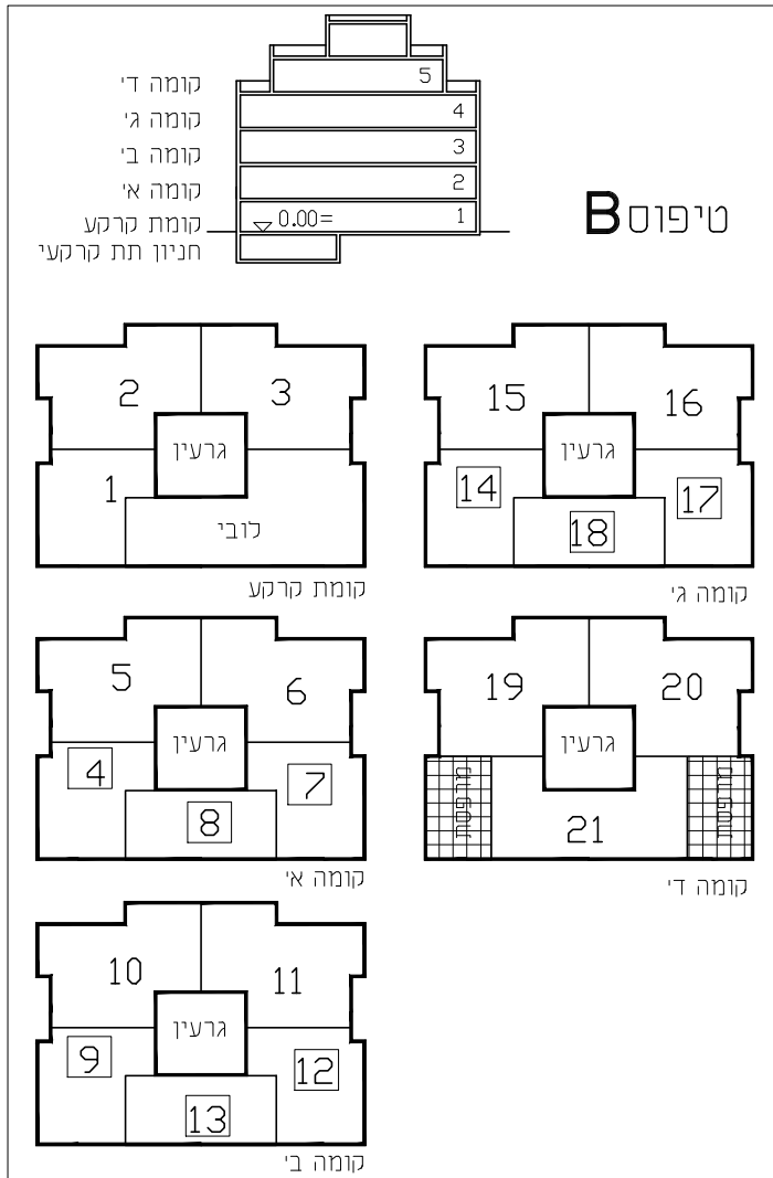
סכמת התפלגות יחיד בבנין מס' 5 בבנין מס' 9
