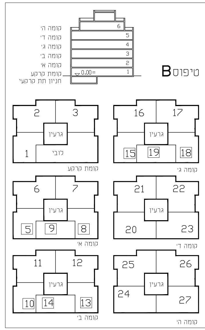
סכמת התפלגות יחיד בנין מס' 23 [9] יחיד קטנות בבנין
