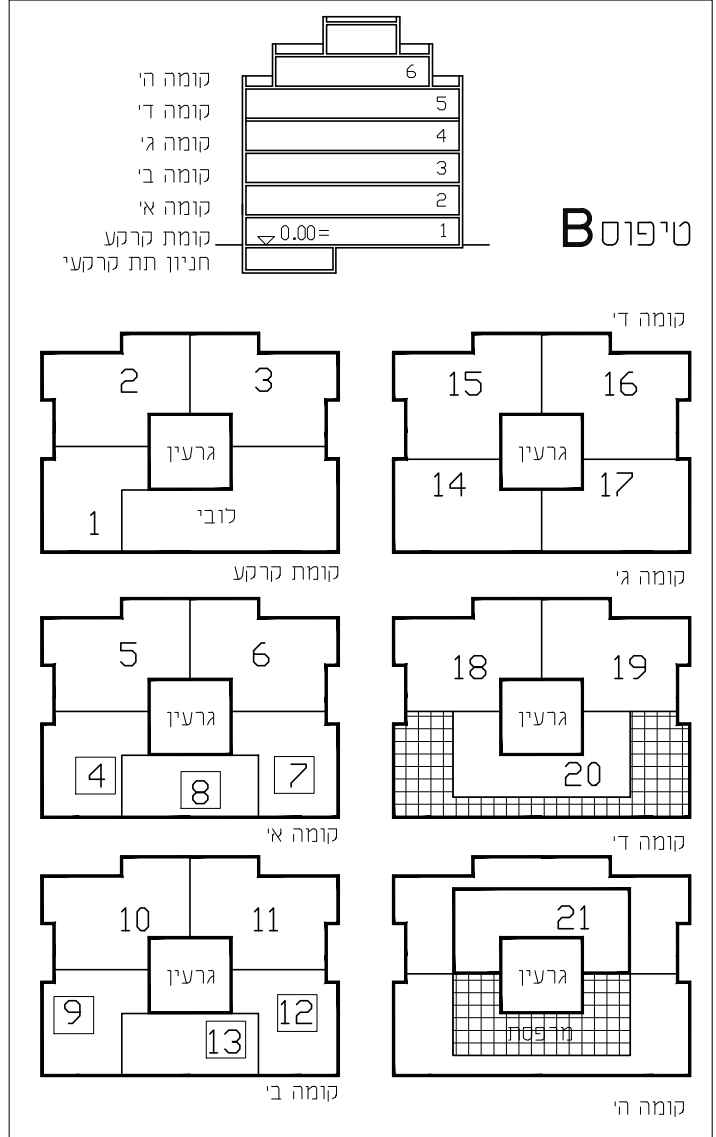
סכמת התפלגות יחיד בנין מס' 37,35 12 יחיד קטנות ב 2 בנינים
