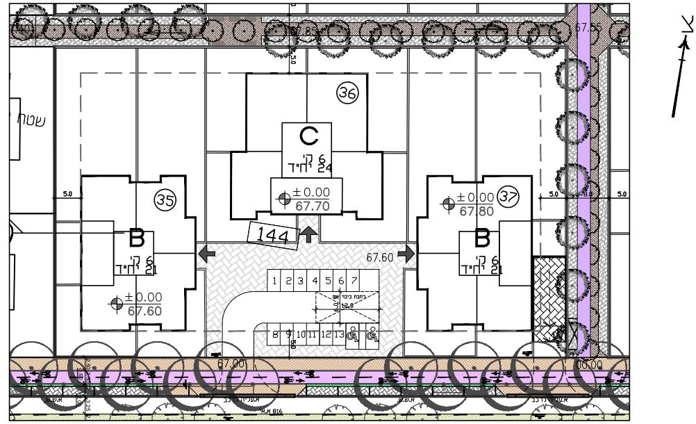
תכנית מגרש מס' 144 ק.מ. 1:1000
